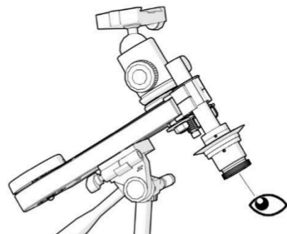
Abbildung 3: So richten Sie die MiniTrack auf den Pol aus
